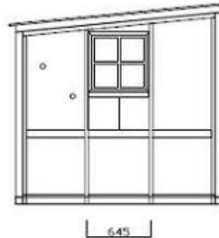
Stomme - syd
