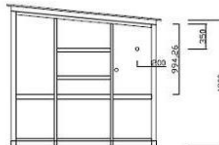
Stomme - norr
