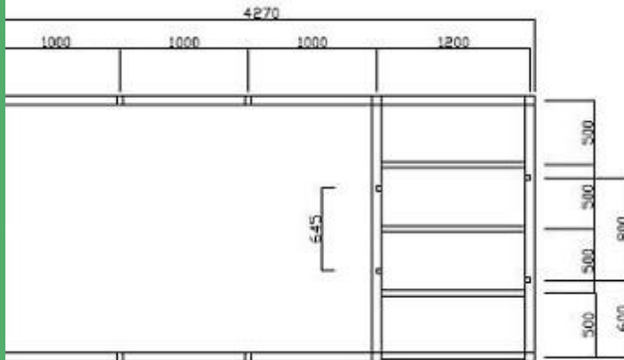
Planritning - stomme
